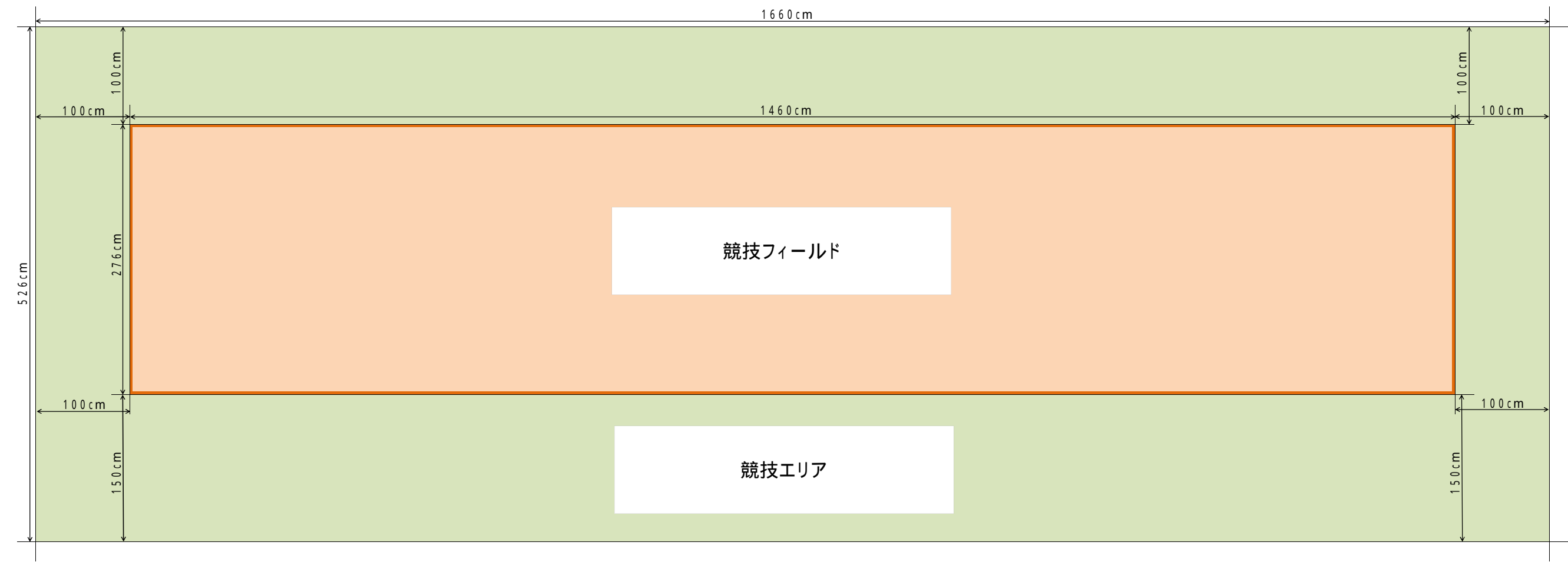
第18回つやまロボットコンテスト 駆け抜ける1300年!!美作国建国ロボコン 競技場図(競技エリア平面図)
