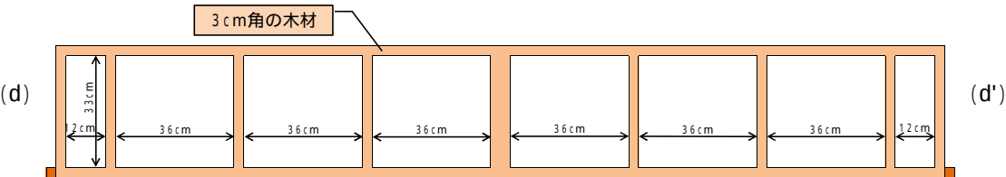
断面(d)―断面(d')
