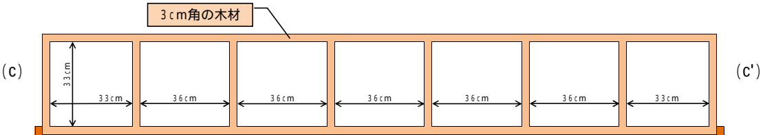
断面(c)―断面(c')
