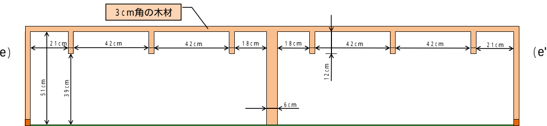
断面(e)―断面(e')
