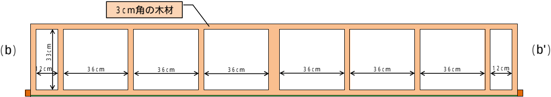
断面(b)―断面(b')
