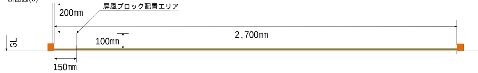
断面図(b)
