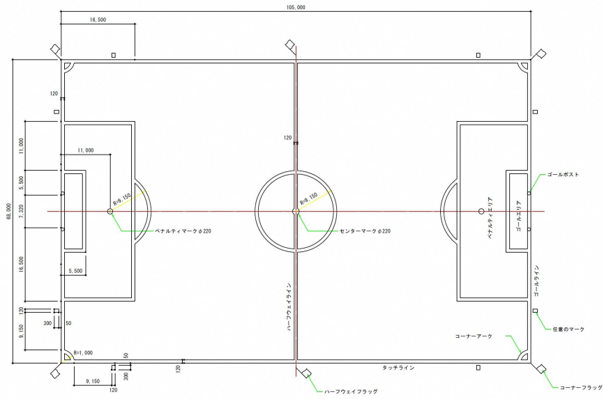
一般サッカーコート ライン図 ラインの幅は120mm、色は白色
