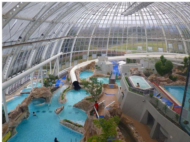
遊泳プール(見下ろし)
