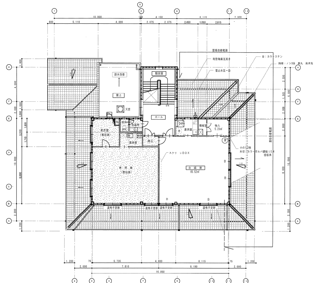
2 階平面図 1/100
