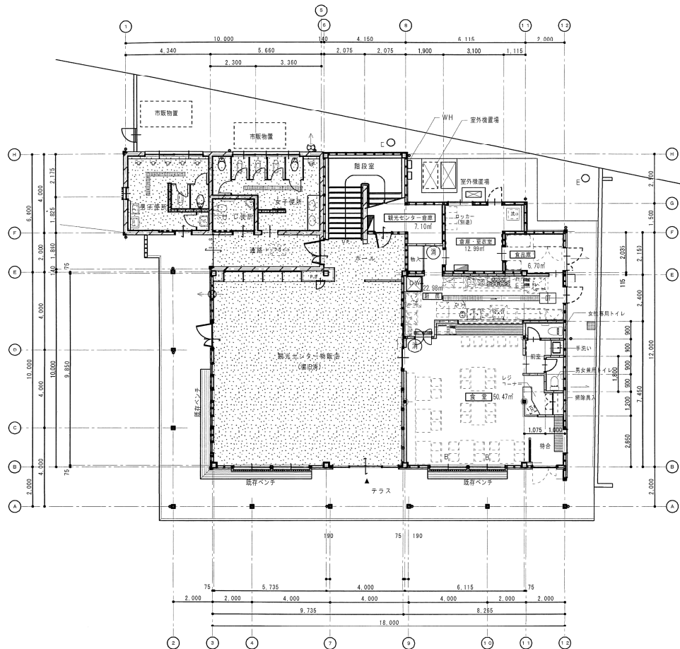
1 階平面図 1/100
