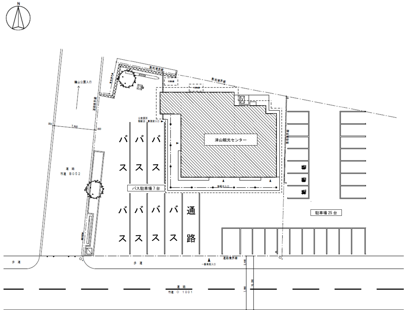
配置図 1/100
