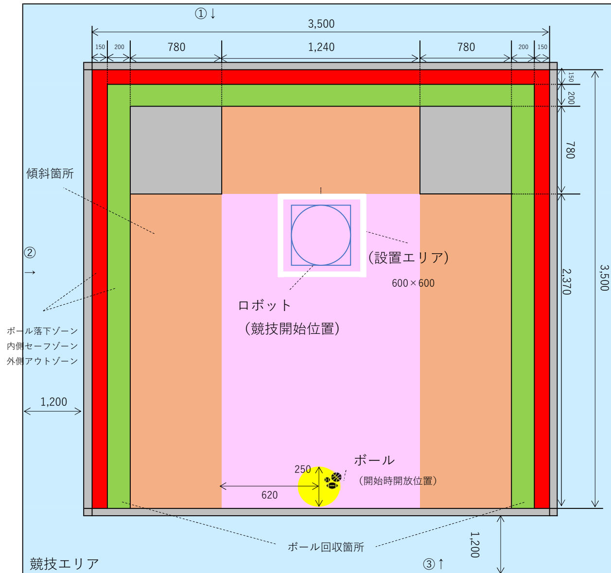
高校一般の部 競技コート図 (平面図)
