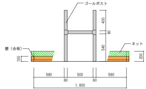
A 立面 (ゴールポスト形状)
