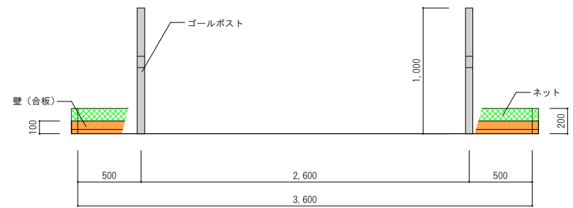
B 立面
