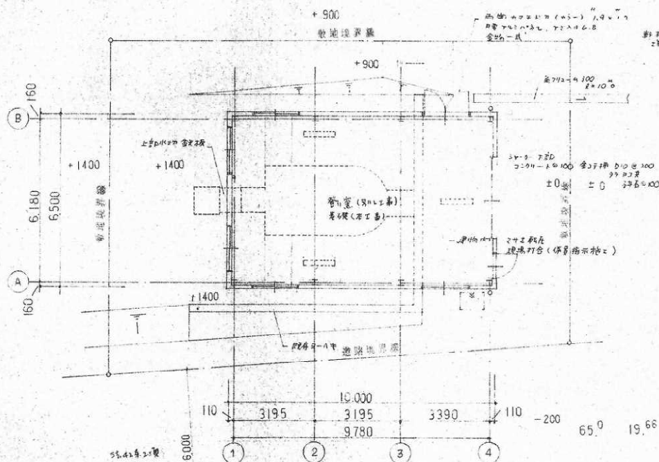
配置図 平面図 \frac{1}{100}
