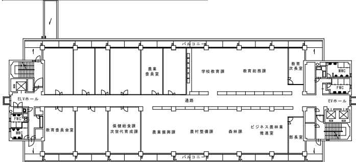
4 階平面図
