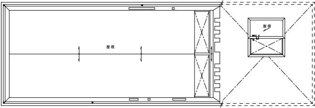
4 階平面図
