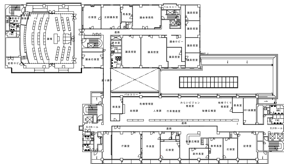
3階平面図
