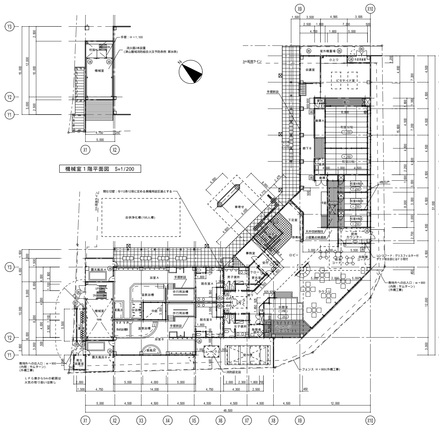
平面図 S=1/200
