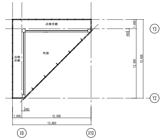
塔屋部平面図 S=1/200
