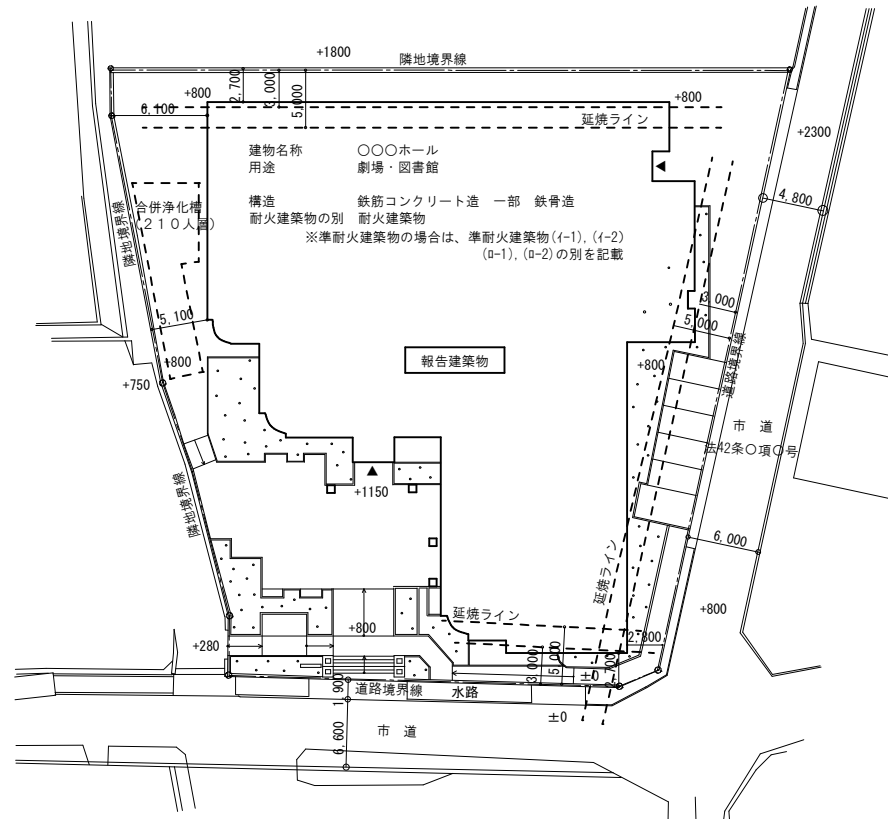
配置図 S=1/800
